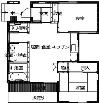
3LDKタイプ 3LDK 面積 A=80㎡ 3~5人以上世帯用
