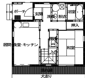
4LDKタイプ 1階平面詳細図
