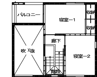
3LDKタイプ 2階平面詳細図
