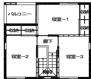
4LDKタイプ 2階平面詳細図
