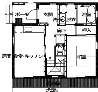
3LDKタイプ 1階平面詳細図
